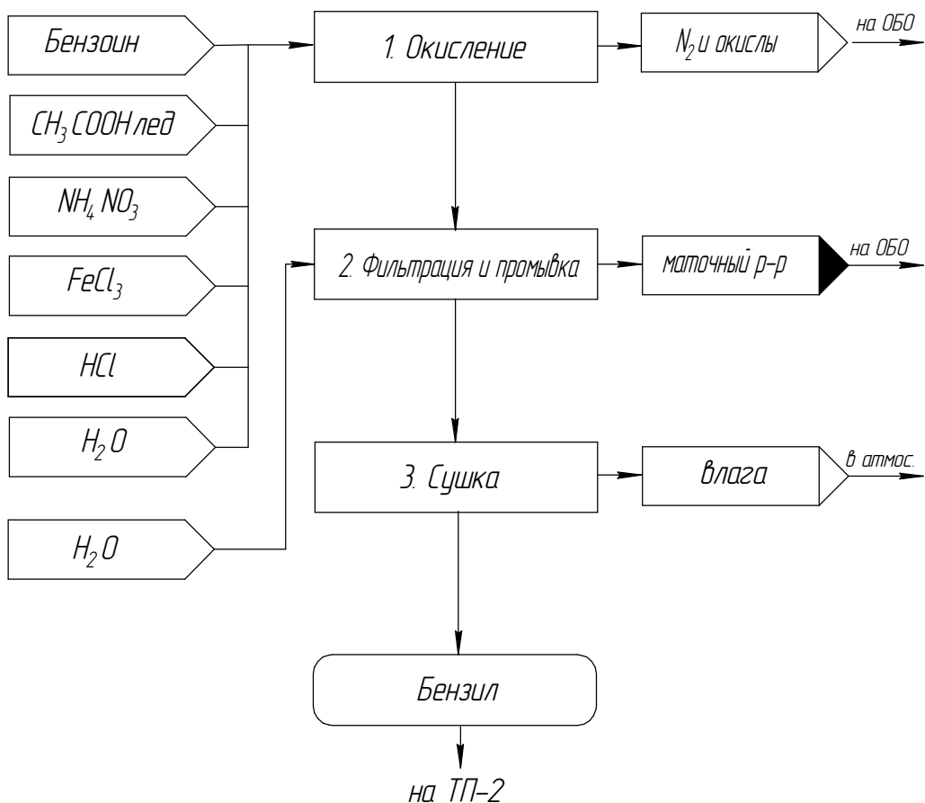
Технологическая схема стадии получения бензила
