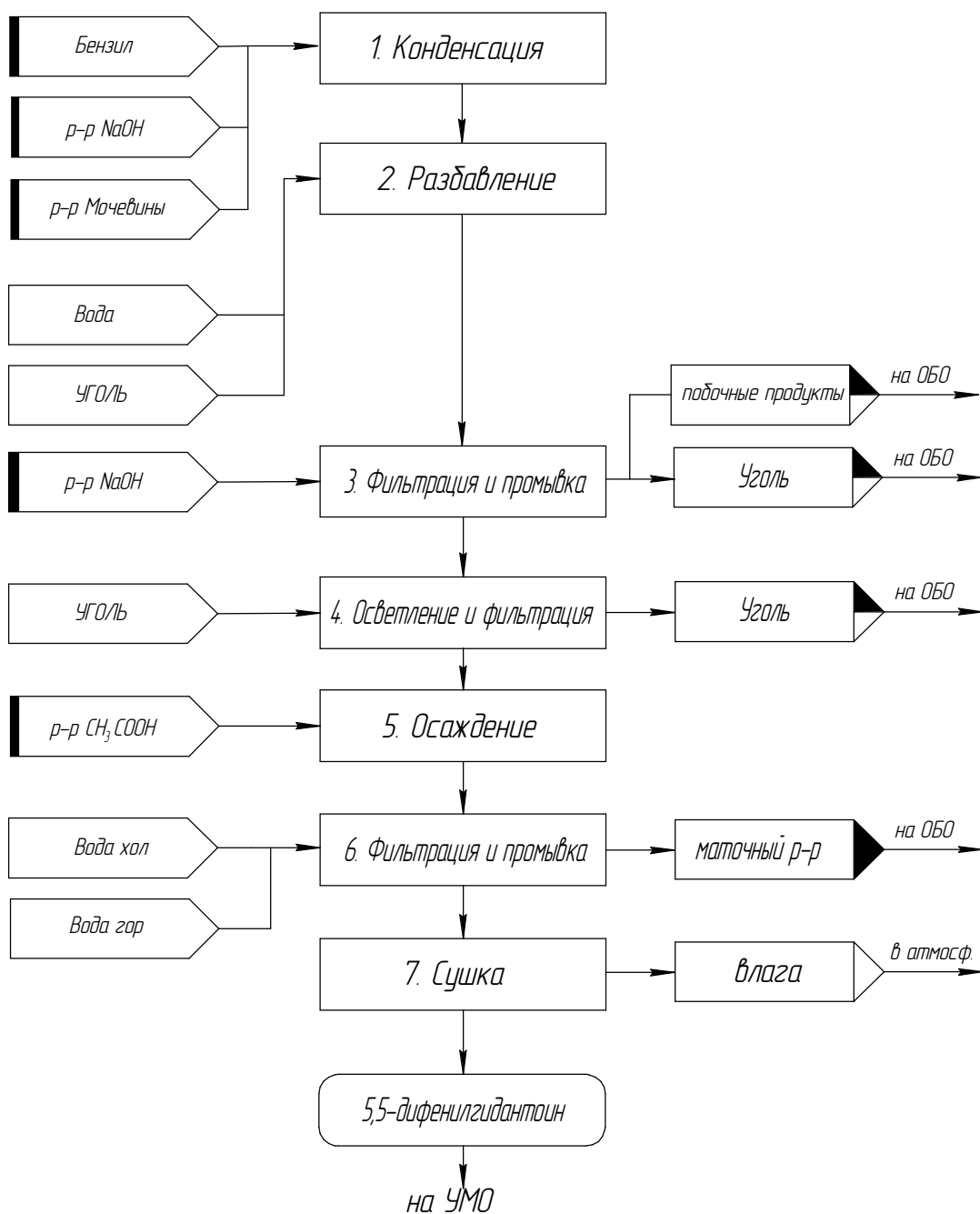
Технологическая схема стадии получения 5,5-дифенилгидантоина
